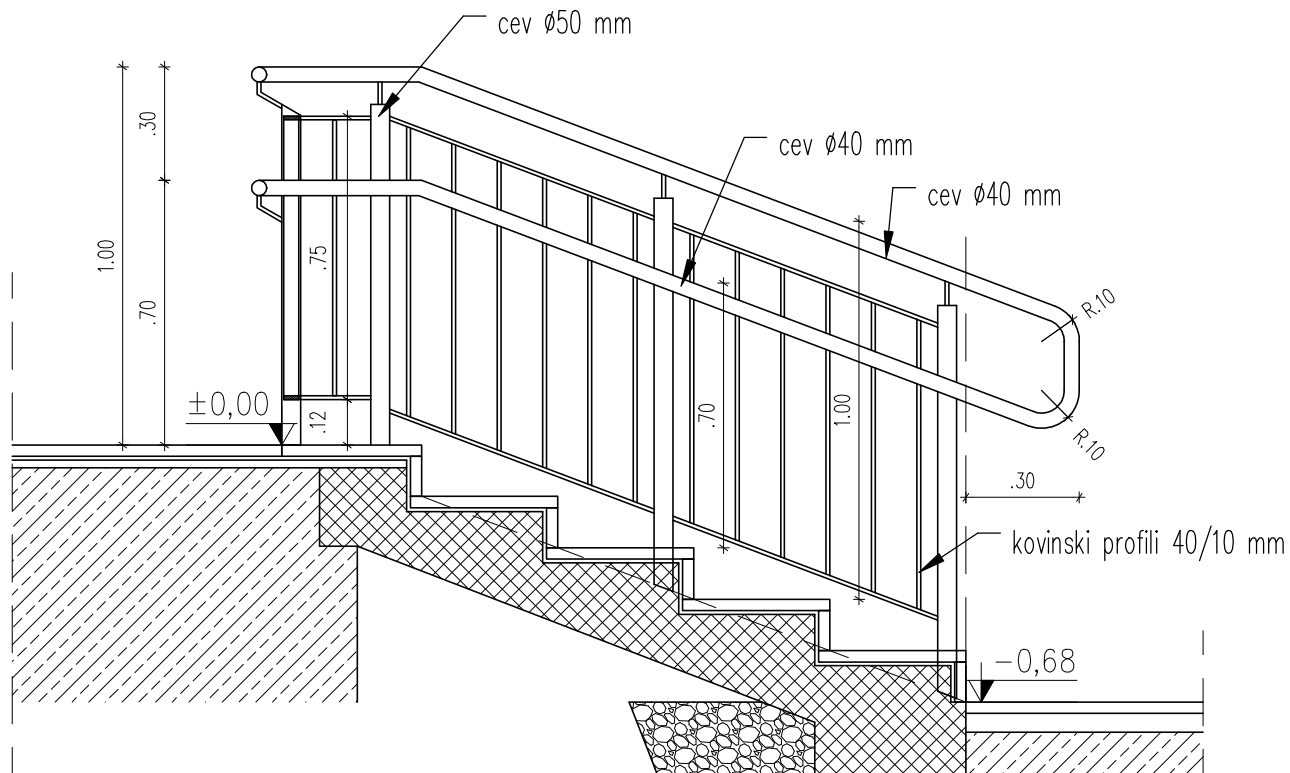
DETAJL STOPNIŠČNE OGRAJE (pogled z notranje strani) M 1:20
